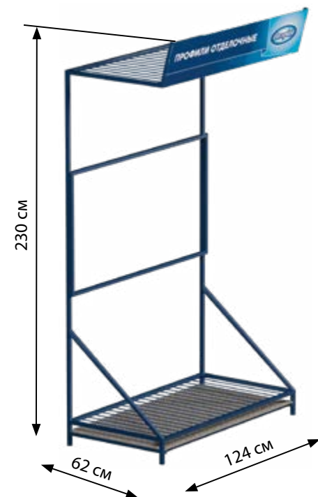
Стенд для профилей 85/12 Decoplast LUX
